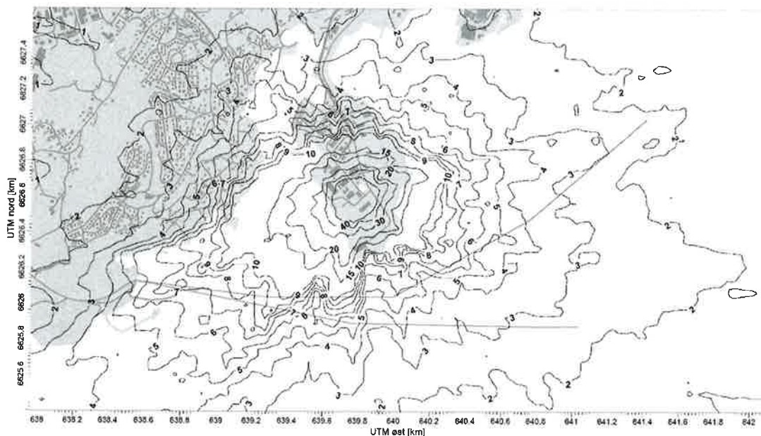
Figur 7 Estimert bidragskonsentrasjon \text{oue}/\text{m}^3 , som årlig 99,7 % timepersentil som estimat for maksimal månedlig 99 % timepersentil ved et utslipp på 50.000 ou/s (forventet worst case).
