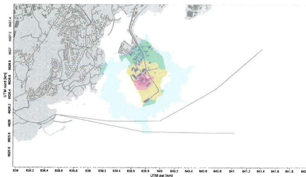
Figur 6 Beregnet luktrisiko (sannsynlighet for overskridelse av timemiddel 1 \text{oue}/\text{m}^3 ) ved et utslipp på 1500 ou/s. RØD : stor risiko (mer enn 1% av timene), ORANSJE : middel til stor risiko (0,5-1% av timene), GUL : liten til middels risiko (0,1-0,5% av timene), GRØNN : liten risiko (0,01-0,5% av timene). Ingen FARGE: svært liten risiko (mindre enn 0,01% av timene).
